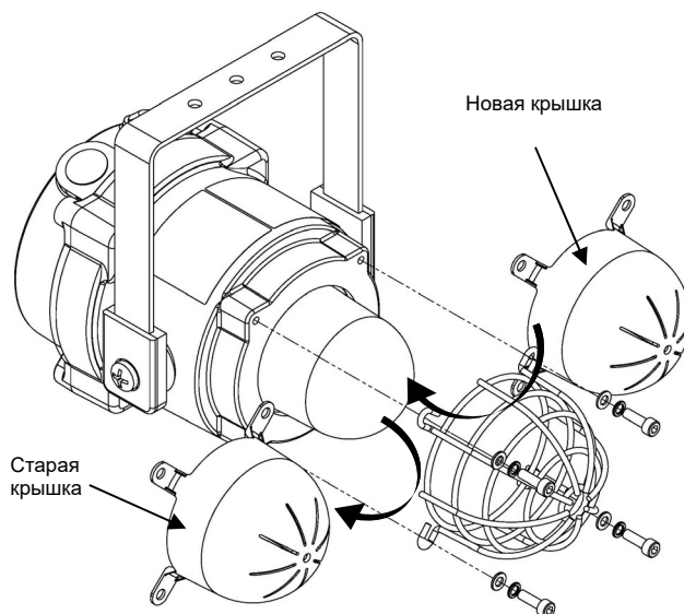
Рис. 12 Замена крышки
