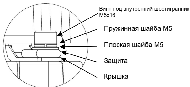
Рис. 13 Порядок крепления крышки и защиты
