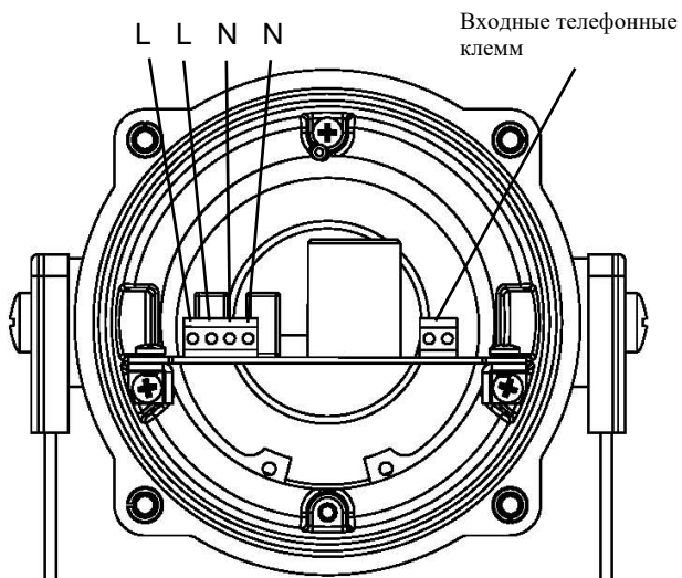
Рис. 6 Клеммы переменного тока
