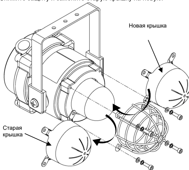
Рис. 12 Замена крышки
