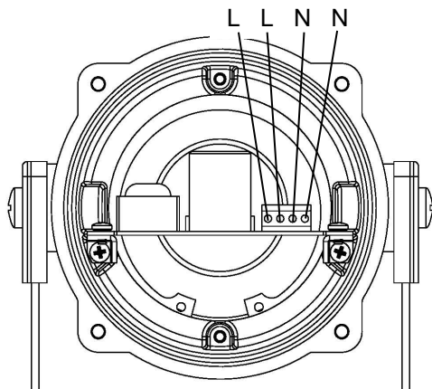
Рис. 6 Клеммы переменного тока
