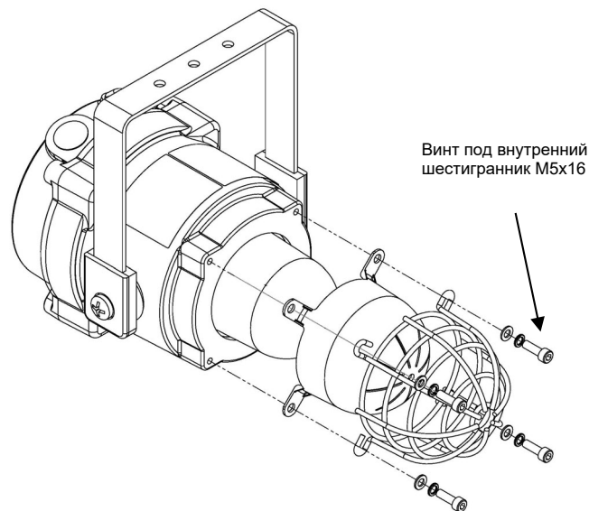
Рис. 11 Снятие крышки
