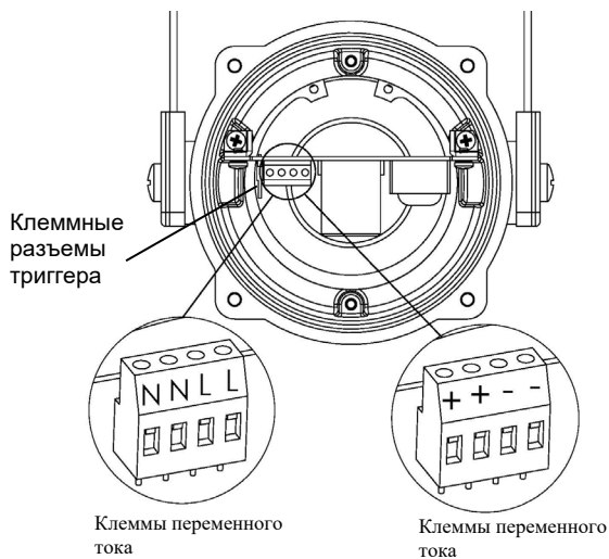
Рис. 4 Внутренний вид маяка VExBGD 5 джоулей
