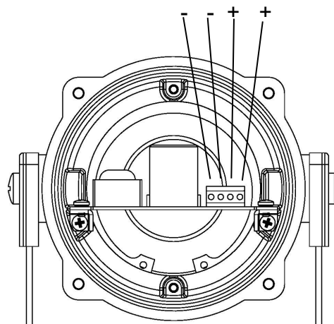
Рис. 8 Клеммы постоянного тока
