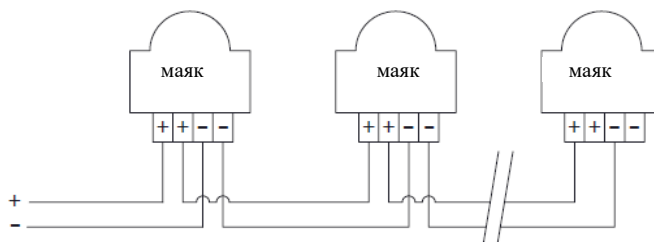
Рис. 7 Упрощенная блок-схема постоянного тока (отрицательное переключение)
