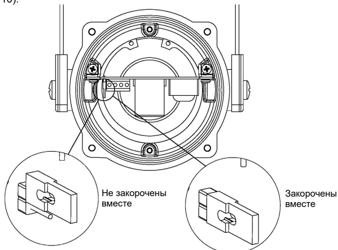
Рис. 10 Настройки разъемов
