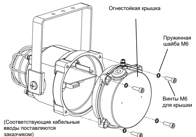
Рис. 2 Доступ к взрывозащищенному корпусу.
