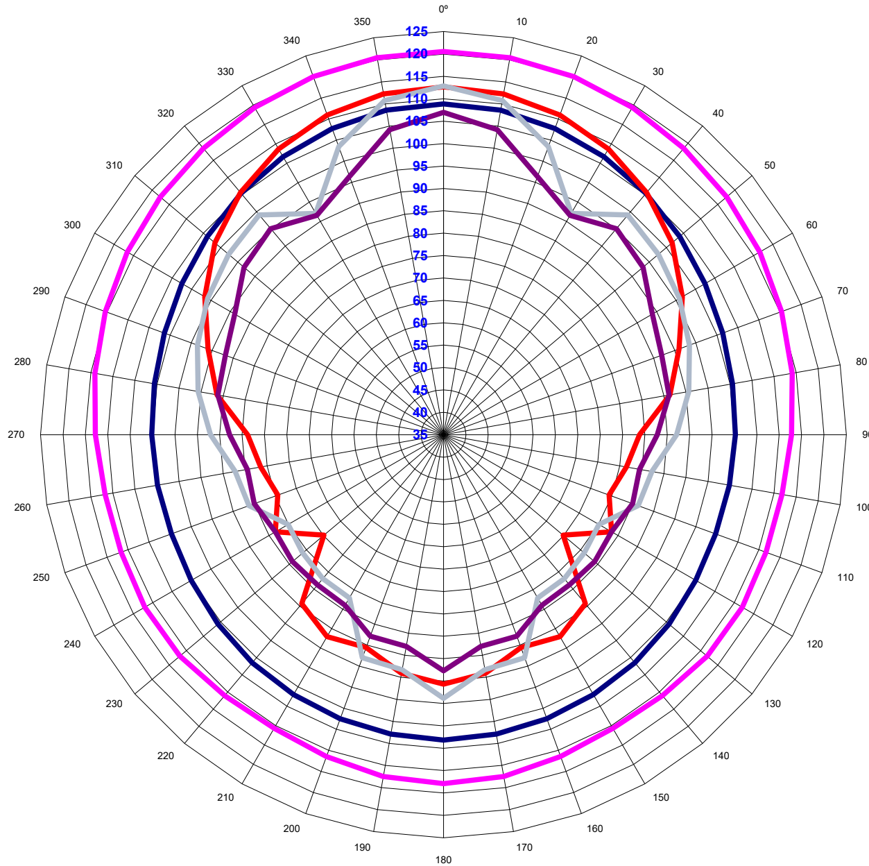
D1xL2F Loudspeaker Polar Plot
