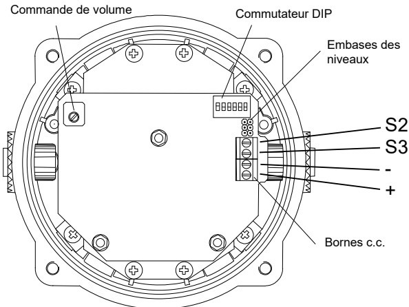
Fig. 6 Bornes c.c.
