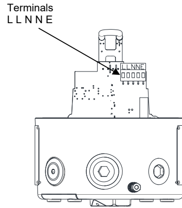
Fig. 4 D1xB2XAC Terminals
