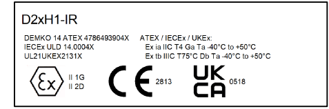
D2xH1-IR Label 3
