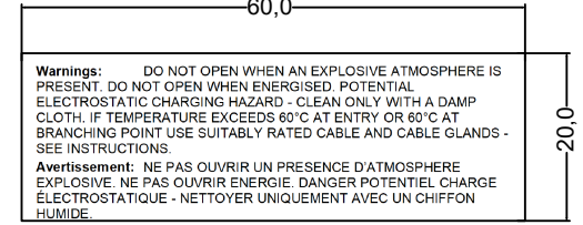
D2xH1-IR Label 2
