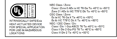
D2xH1-I Label 4
