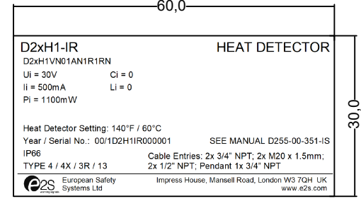
D2xH1-IR Label 1
