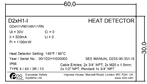
D2xH1-I Label 1
