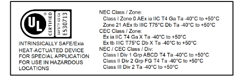
D2xH1-IR Label 4
